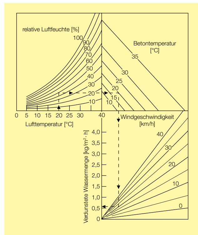
Bild 1: Das Austrocknungsverhalten von Beton in Abhängigkeit von Windgeschwindigkeit, Luftfeuchtigkeit und Temperatureinfluss [4]
