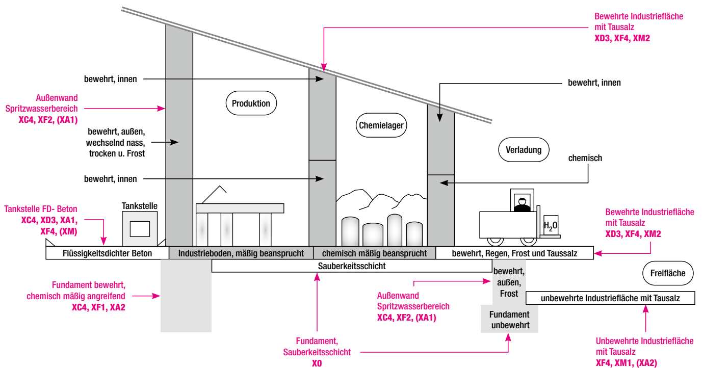
Beispiele für mehrere, gleichzeitig zutreffende Expositionsklassen im Hoch- und Ingenieurbau
