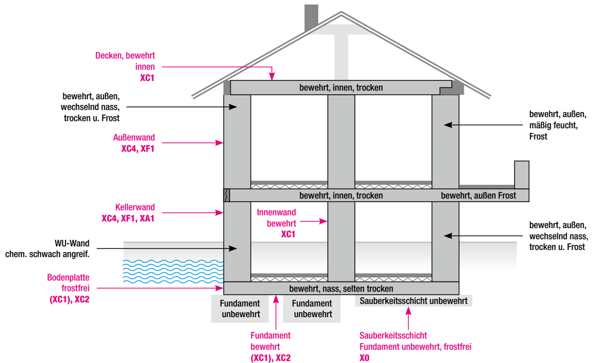
Beispiele für mehrere, gleichzeitig zutreffende Expositionsklassen an einem Wohnhaus
